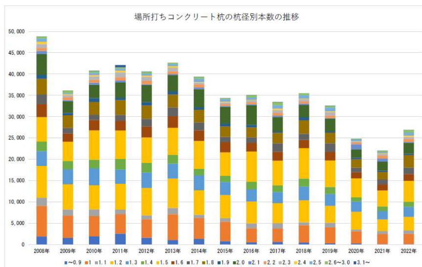
図 2.10 場所打ちコンクリート杭 年代別 杭径の推移 (本)
