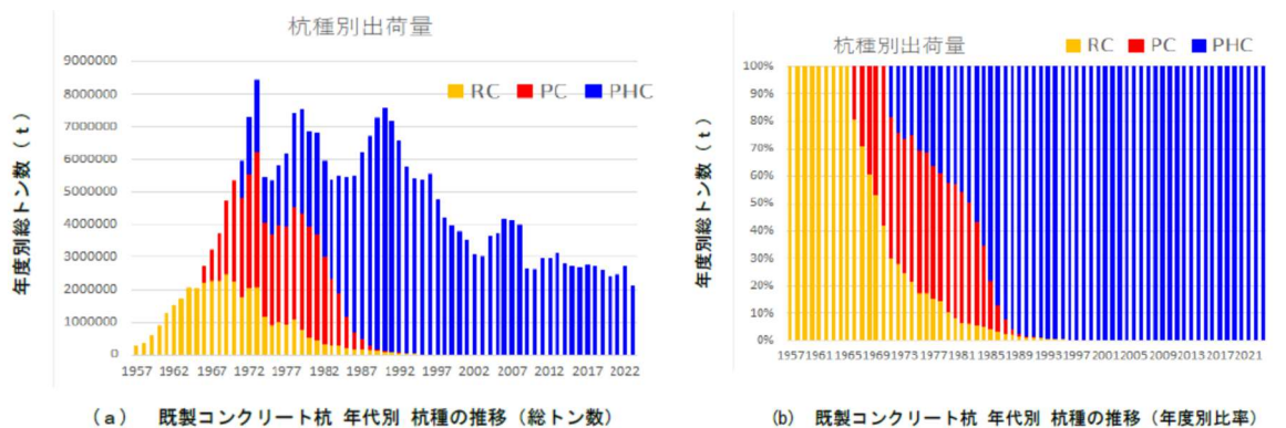
図 2.6 既製コンクリート杭 年代別 杭種の推移（年度計）
