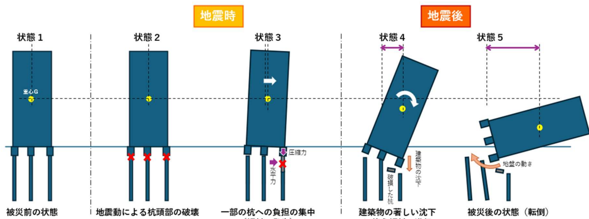
図1.1 地震により転倒被害を生じた建築物の転倒シナリオ 1)
