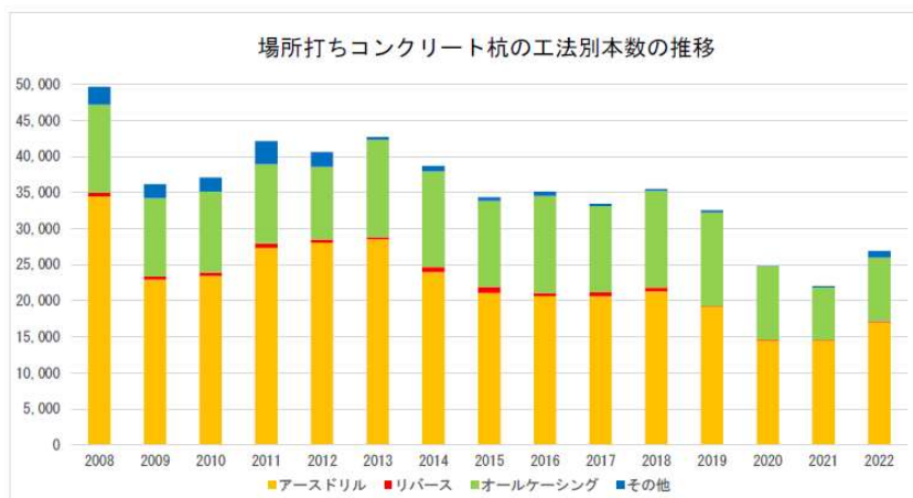
図 2.9 場所打ちコンクリート杭 年代別 杭本数の推移 (本)
