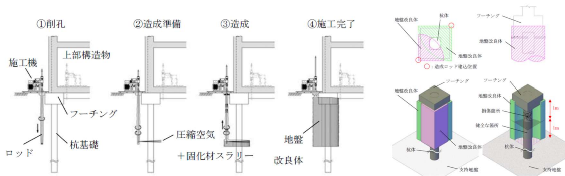
図 3.5 地盤改良（高圧噴射）による杭頭の補強 2 3)
