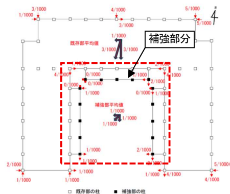
(b) 平面図
