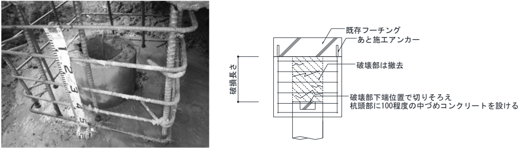
図 3.3 パイルキャップの増し打ちによる杭頭の補強 21)
