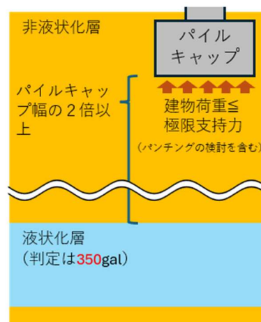
図 2.5 パイルキャップ直下に一定の非液状化層が存在する場合
