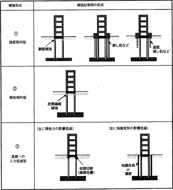
図 3.2 杭基礎の耐震補強工法の例
