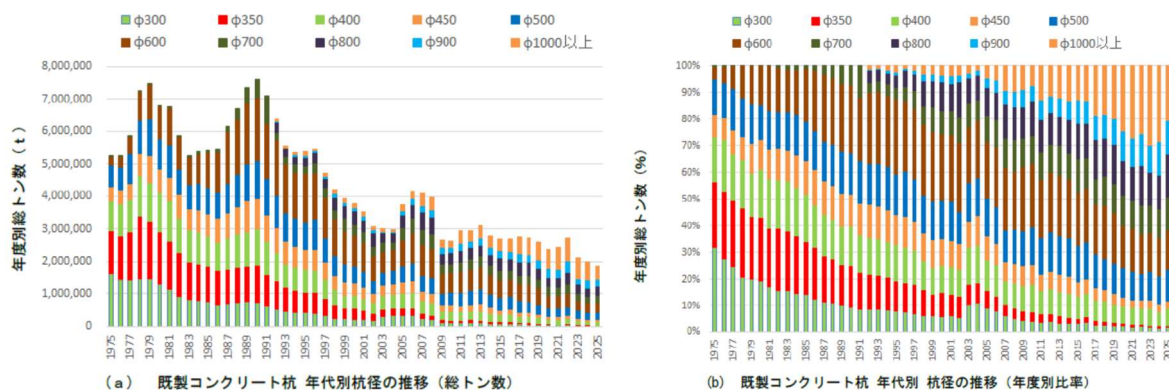
図 2.7 既製コンクリート杭 年代別 杭径の推移（年度計）
