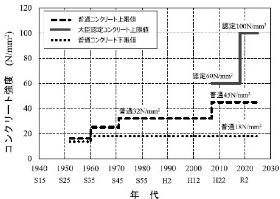
図 2.11 場所打ち杭のコンクリート強度の上限値と下限値の推移 1 7)
