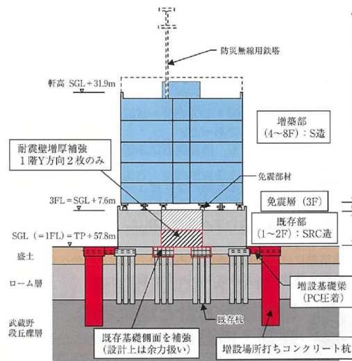
図 3.7 増し杭による補強 20)
