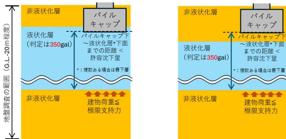
(a) パイルキャップ直下が液状化層の場合 (b) パイルキャップ直下が非液状化層の場合
