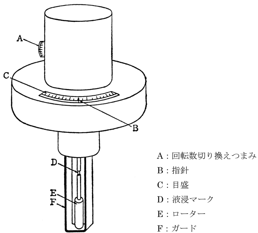
図 2 回転粘度計
