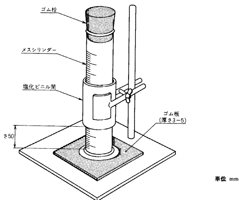
見かけ比容測定器の一例（タップ法）
