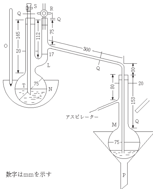
図2 減圧蒸留装置
