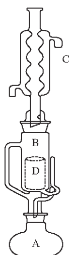
A : フラスコ B : 抽出管 C : 球管冷却管 D : 円筒ろ紙
