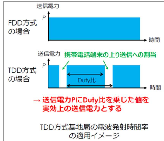
図11 TDD方式基地局の電波発射時間率の適用イメージ ( F_{\text{TDC}} の参考)
