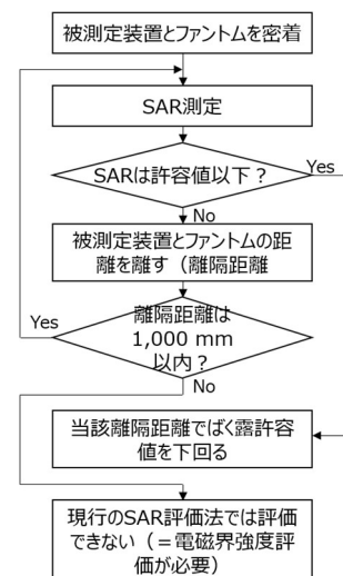
図4 被測定装置とファントム間の離隔距離に着目した測定フロー
