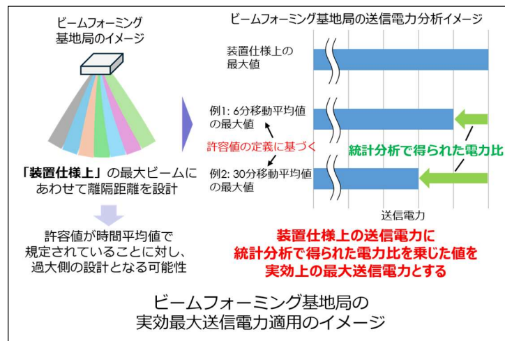
図12 ビームフォーミング基地局のActual maximum approachの適用イメージ ( F_{\text{PR}} の参考)
