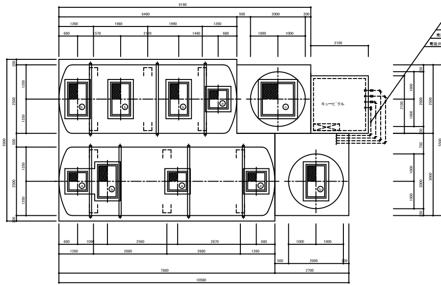
上部平面図 1/50
