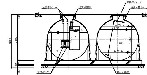
D-D断面図 1/50
