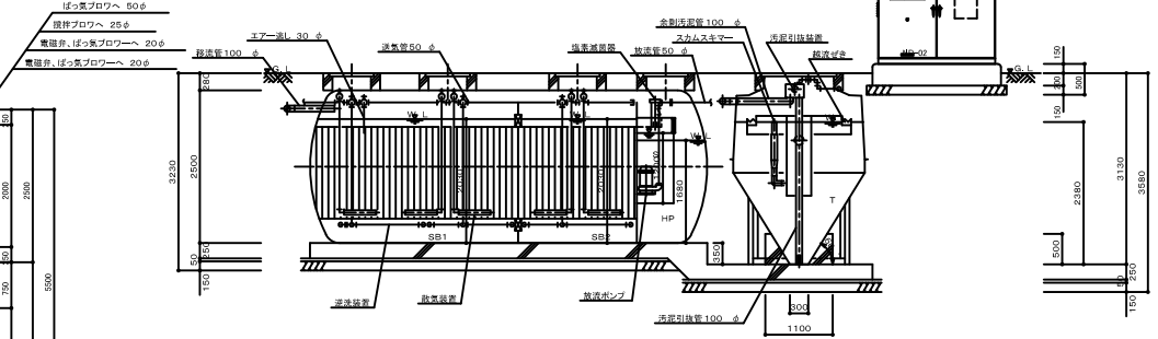
A-A断面図 1/50
