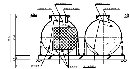
C-C断面図 1/50
