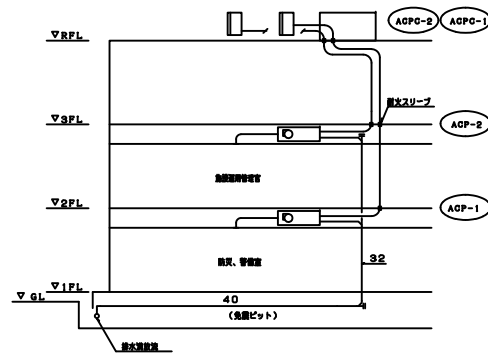
業務棟ルームエアコン配管
