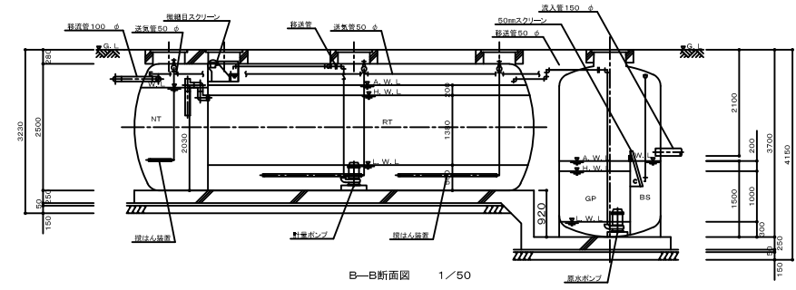
B-B断面図 1/50
