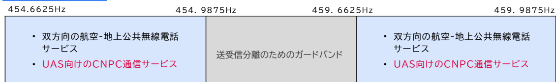
図 31 450-470 MHz 帯におけるチャネルプラン 42
