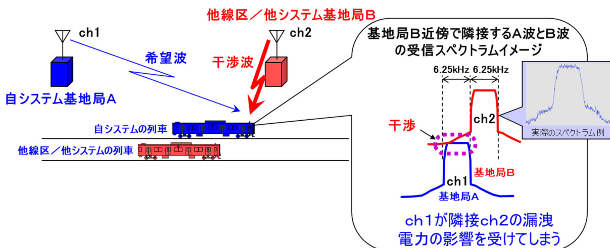
図 2-4 隣接チャネル干渉のイメージ
