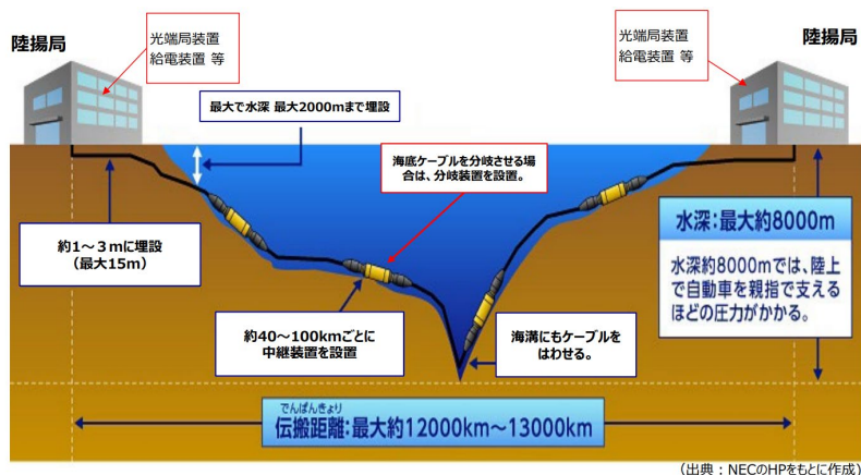
図表1ー1 海底ケーブルシステムの全体像(構成例)
