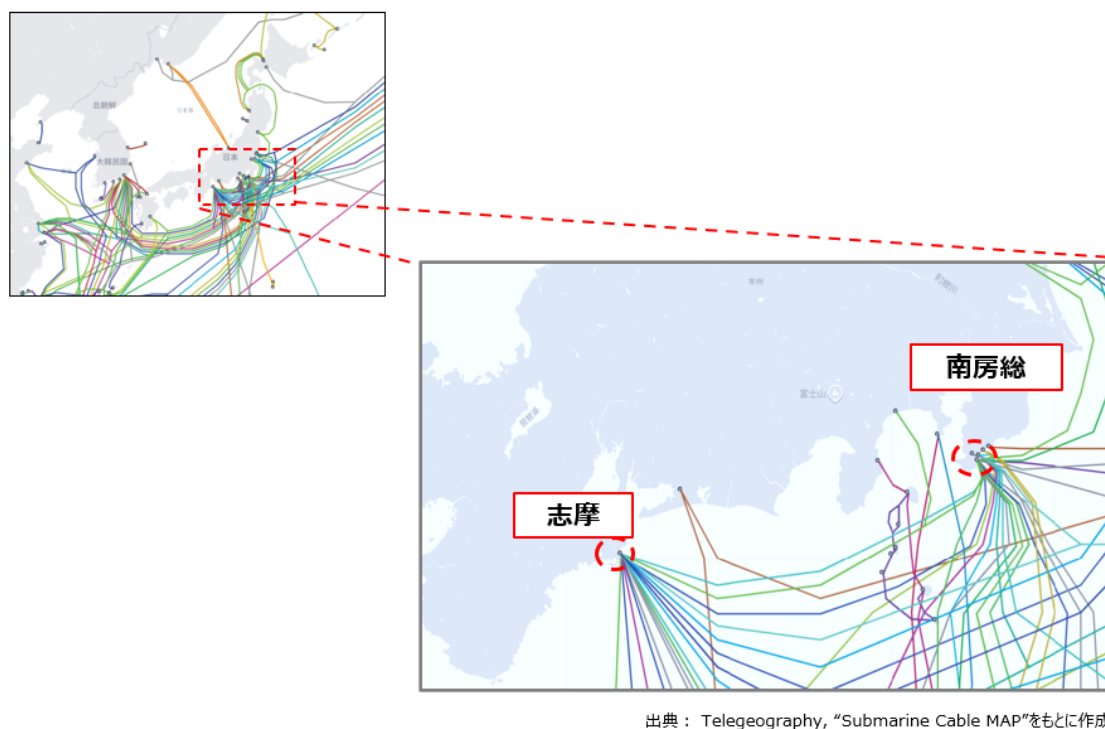
図表2—2 我が国の国際海底ケーブルの陸揚局の実態
