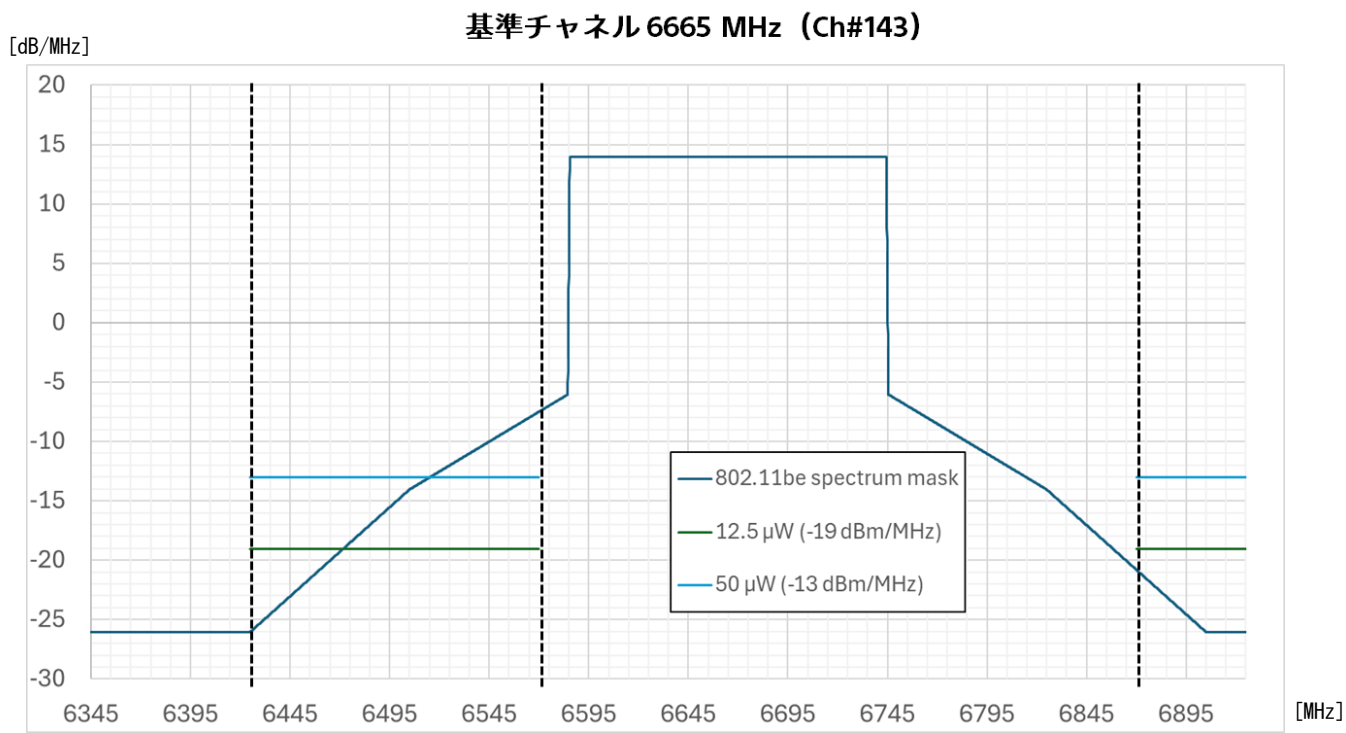
図 2-29 : 160 MHz BW の場合 (6870 MHz 超の領域)
