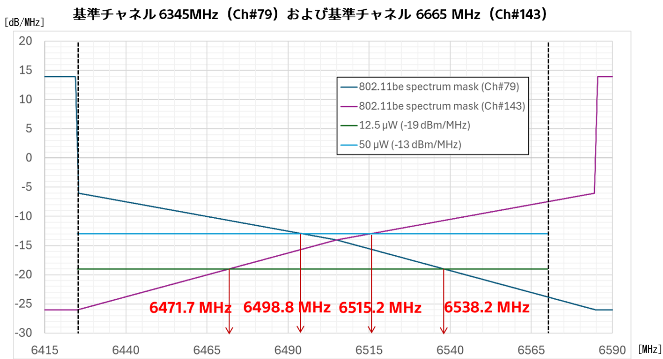
図 2-28 : 160 MHz BW の場合 (6425 MHz 超 6570 MHz 未満の領域)
