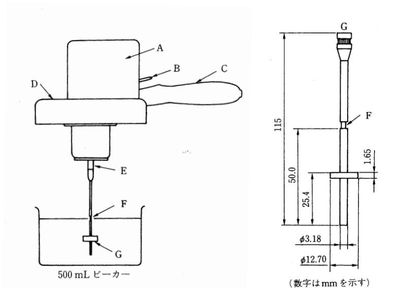
ブルックフィールド型粘度計
