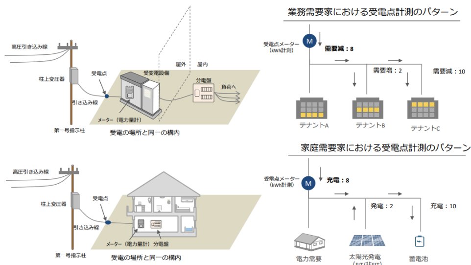
図6 受電点計測のイメージ
