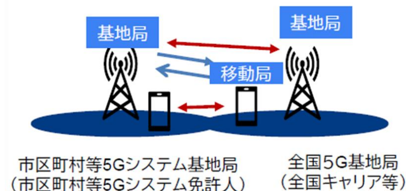
図 2. 1-20 26GHz 帯 5Gシステム相互間の検討（隣接周波数：非同期運用）<シナリオ2>
