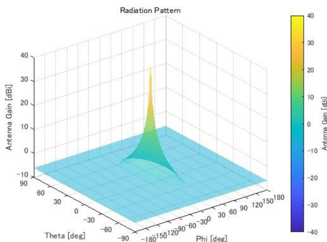
図 2. 2-3 40GHz 帯 FPU の空中線指向性
