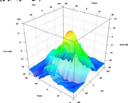
(最大パターン)
