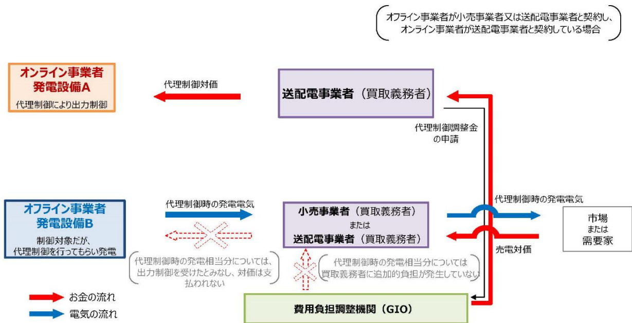
【図表 1110】 オンライン代理制御のスキーム
