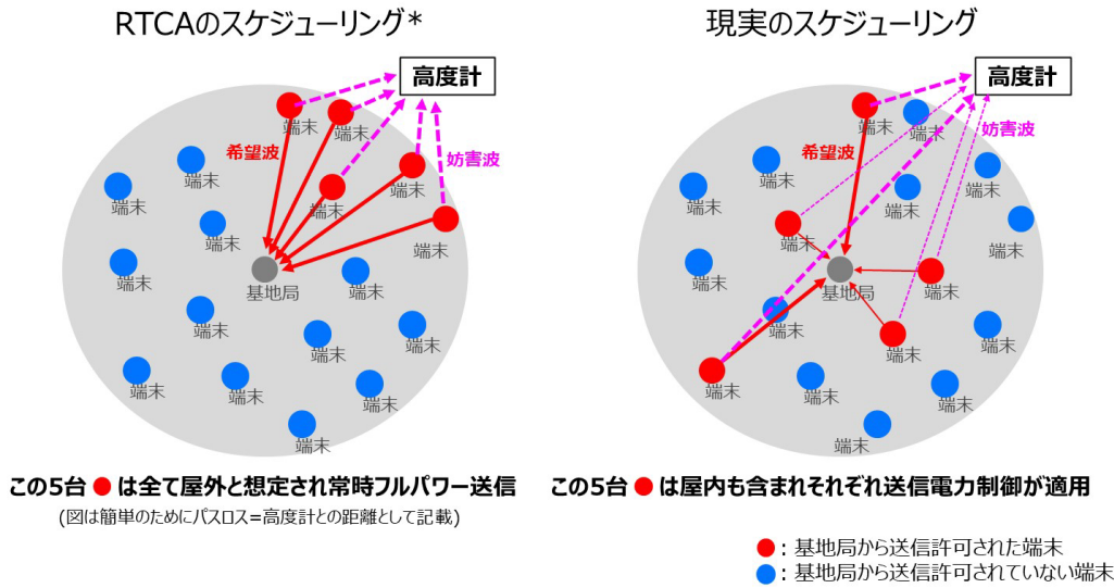
図3. 4. 2-4 基地局との間で通信を行うために実際に電波を発射する HPUE が選択される (スケジューリング) 条件
