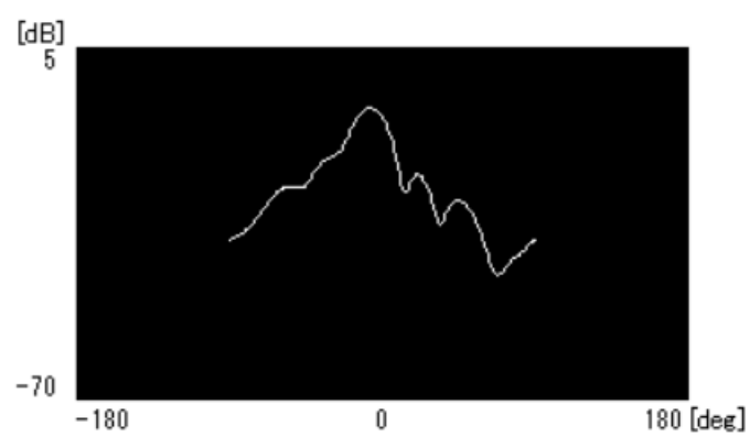
図 4. 2 - 3 PC 1 端末平均パターン
