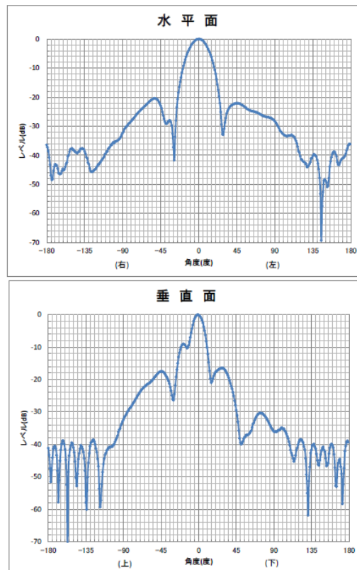
図 3. 5. 1-1 5GHz 帯無線アクセスシステムの空中線指向特性
