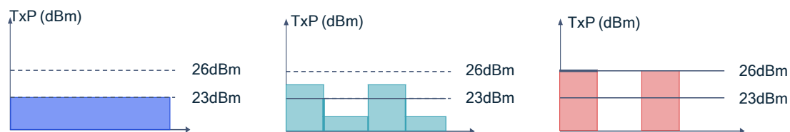
図 1. 2. 2-1 空中線電力の時間的な変化例
