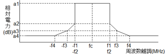
図1 送信信号特性
