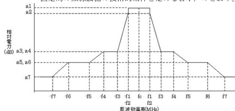
図 送信スペクトルマスク
