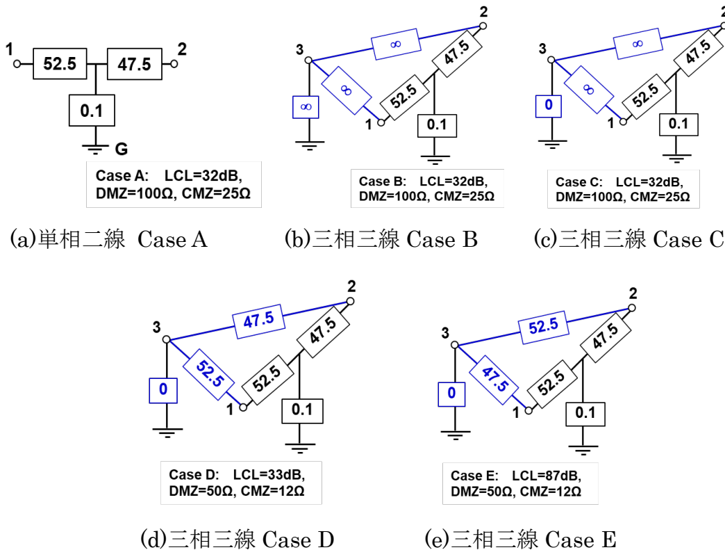
図 5.9 PLC 設備接続 2 線と第 3 線との接続条件を変えた解析モデル (PLC 設備接続 2 線の平衡状態が良い場合。図の数字は抵抗値 Ω)
