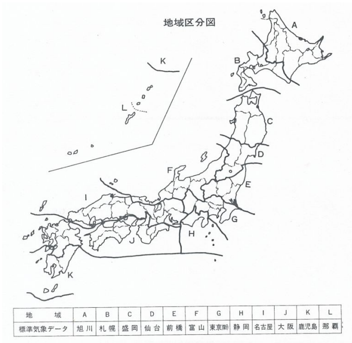
図2 地域区分図
