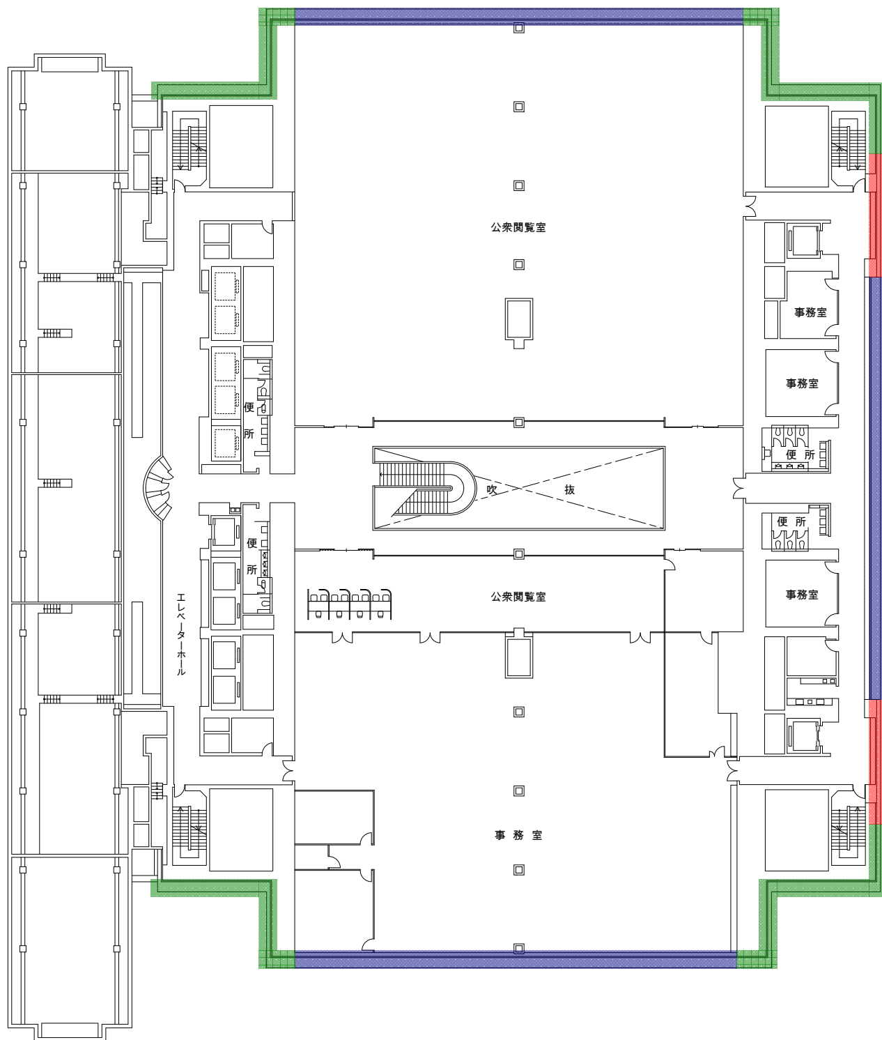
2階平面図
