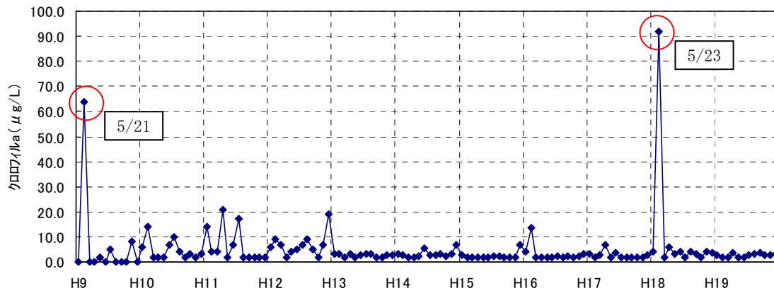
図 6.8 弥栄ダムのクロロフィル a の推移
