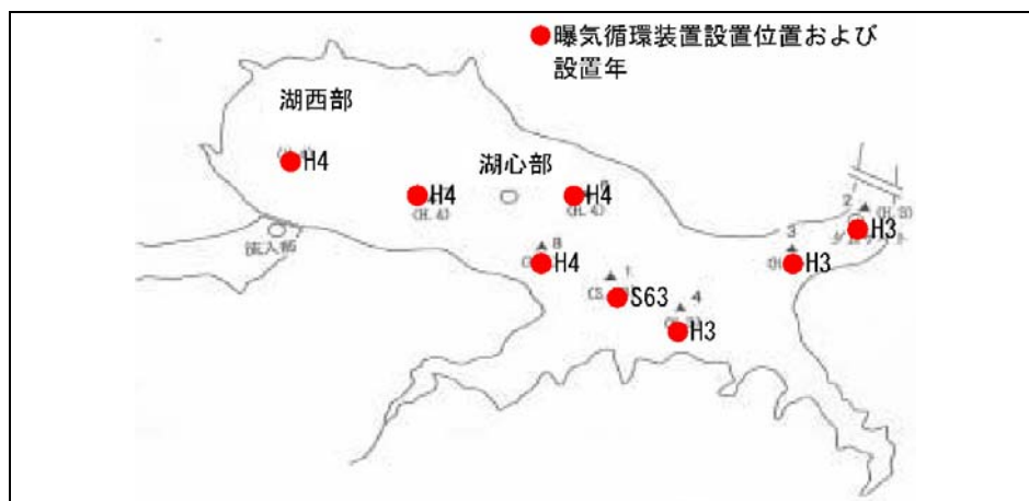
図 3.7 相模ダム（相模湖）曝気循環装置設置位置
