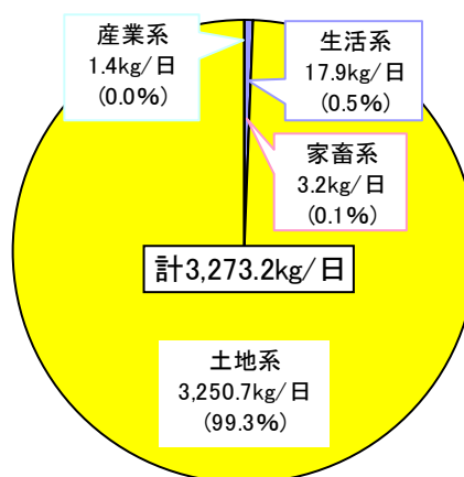
川治ダム(COD): 将来・平成25年度
