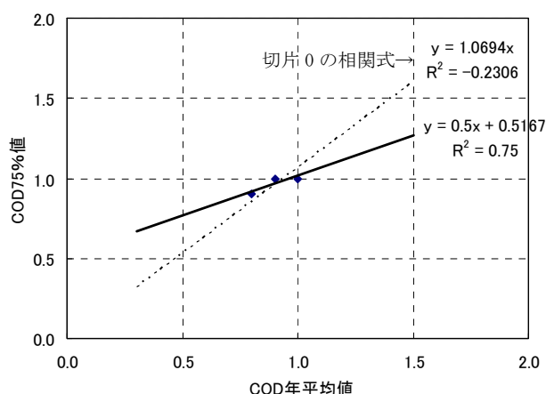
深山ダム COD年平均値と75%値 平成15年度~平成17年度
