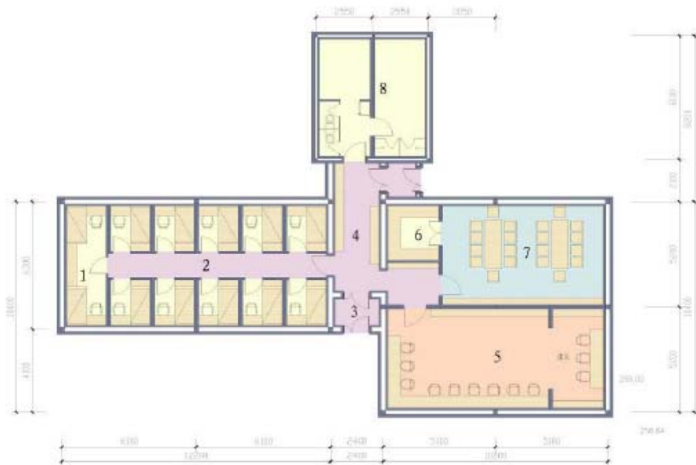
図6 中心建築物内部
