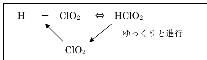
図 2. 弱酸性領域での酸性 \text{ClO}_2^- 、 \text{HClO}_2 及び \text{ClO}_2 間サイクル反応の持続（参照 3）
