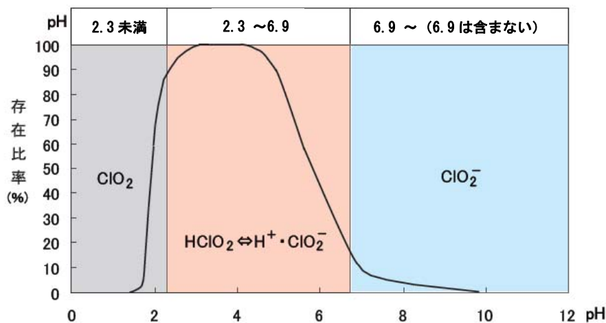
図 1 亜塩素酸水に含有する塩素酸化物の pH による存在比の変化（事業者提供資料より）
