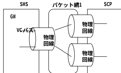
図3.1 ネットワーク構成 (PHS)
