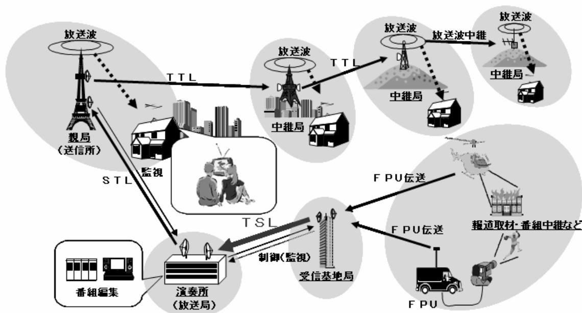
図 1-3 監視・制御用固定回線の例
