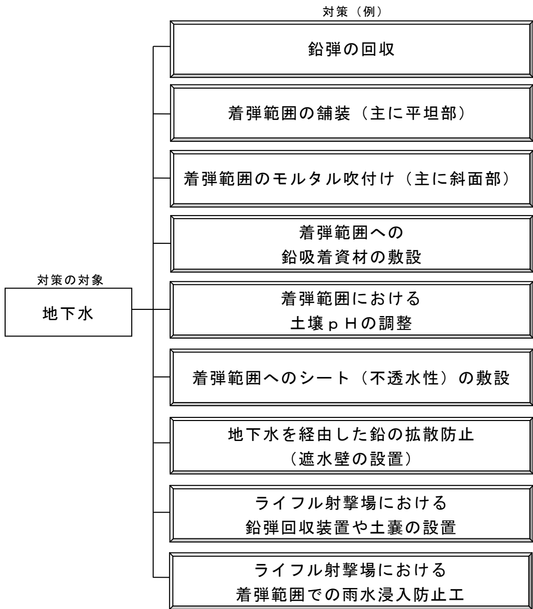
図３－３ 鉛汚染問題の解消を対策目的とした場合の対策の例② （地下水を対策の対象とした場合）
