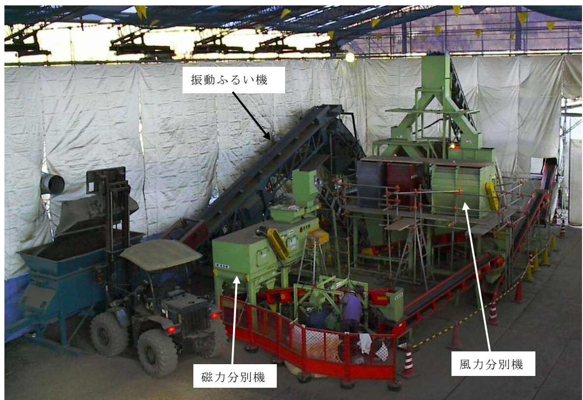
図 5－2 分別機等を用いた作業状況の例
