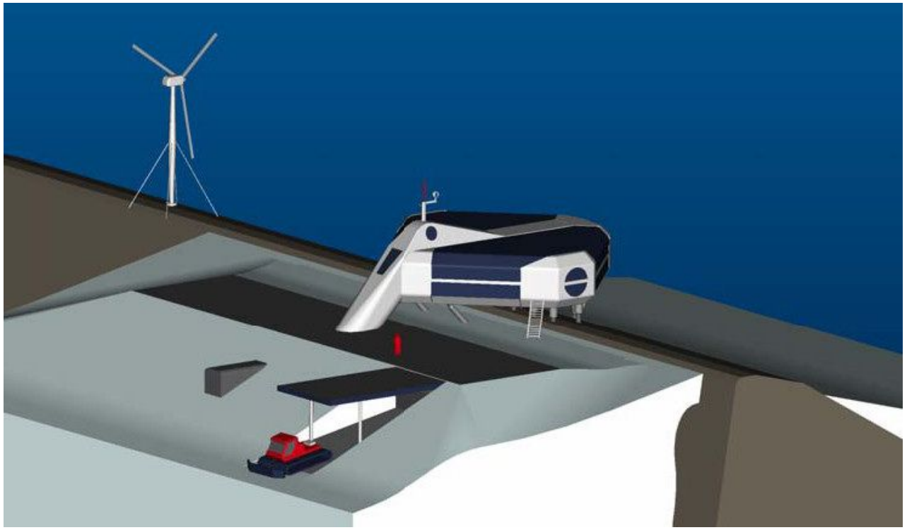
図4 基地立体図
