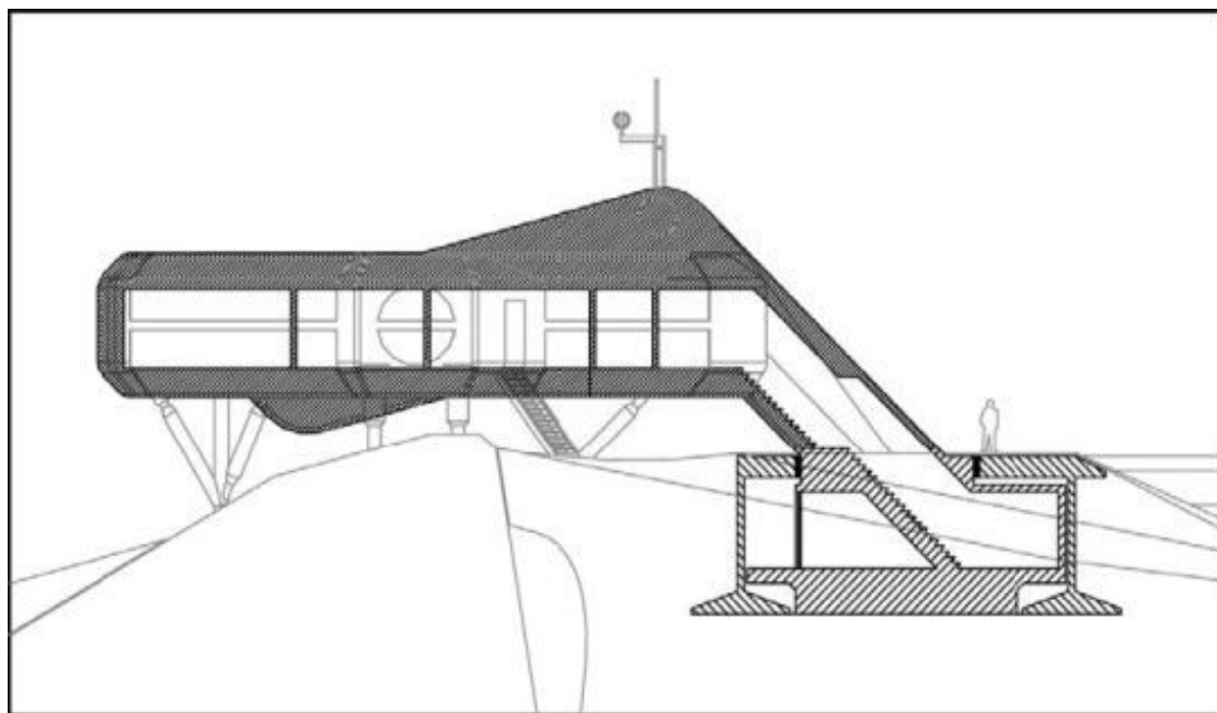
図7 基地断面図
