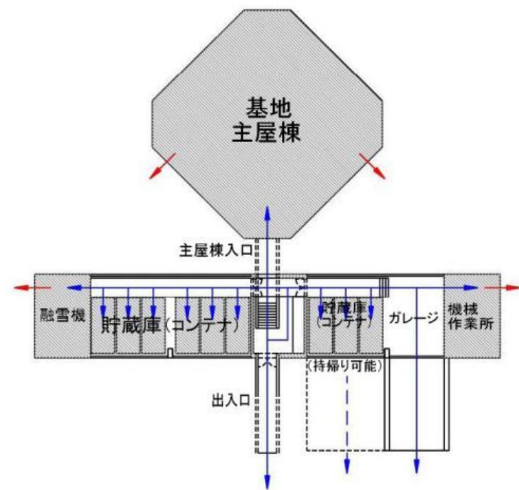
図6 倉庫 / 貯蔵棟平面図
